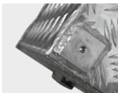
An der Unterseite 4 Füße mit Innengewinde M10 für dauerhafte Befestigung
