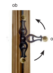
Maniement de l'espagnolette en sens antihoraire
