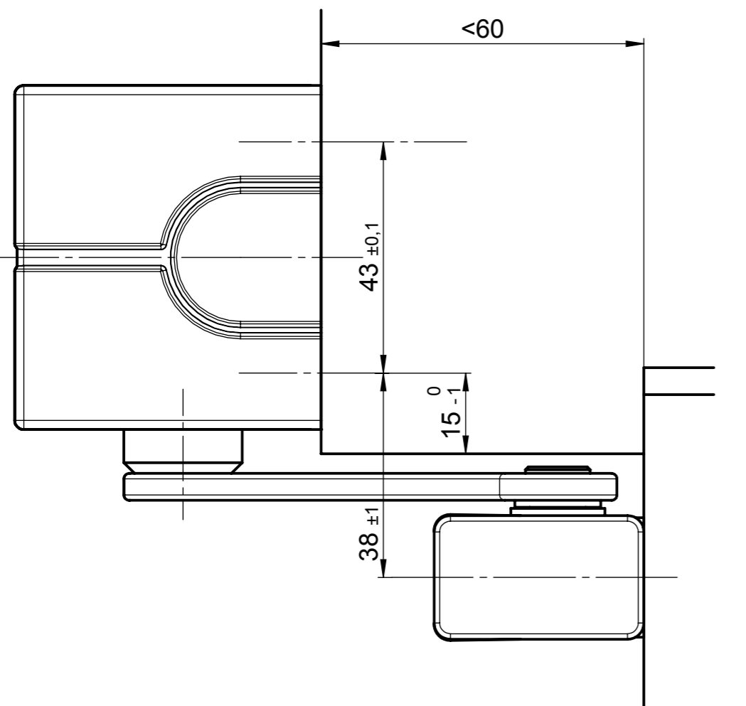
DIN rechts right hand door
