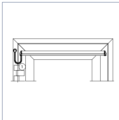
Sicherheitssensor „Offen“ auf der Bandseite montiert
