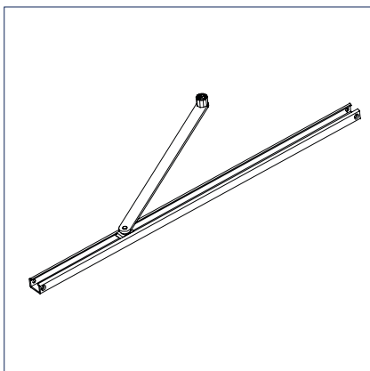
Rollen- / Gleitschiene mit Hebel
