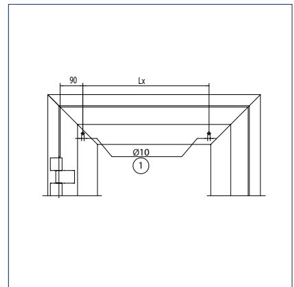
Sicherheitssensor Lochbild Bandseite
