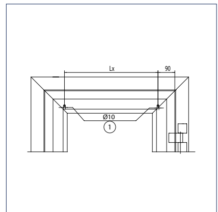
Sicherheitssensor Lochbild Bandgegenseite
