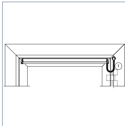
Sicherheitssensor „Schließen“ auf der Bandgegenseite montiert
