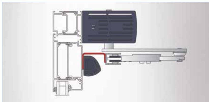
Adapter für Sensor und Gestänge für Slimdrive EMD und TSA 160 NT
