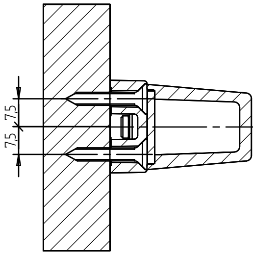
SCHNITT A-A
