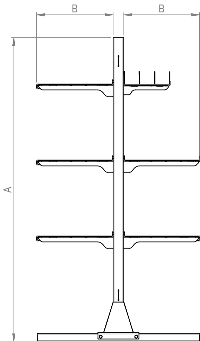
Totale Säulenbelastung für doppelseitige Säule und Boden- Deckensperrsäule
